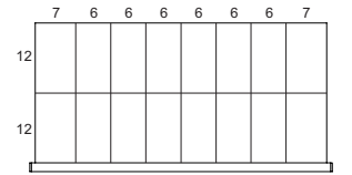
R_JG-A0708__ 16 COMPARTIMIENTOS
