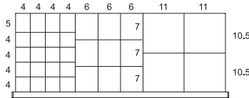
R__KE-D0824__ 33 COMPARTIMIENTOS
