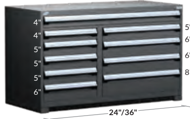
10 CAJONES R5KKE-3403 60" x 24" x 36" R5KKG-3403 60" x 27" x 36"
