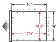
ANAQUEL DESLIZABLE LATERAL
