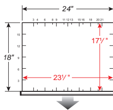
MEDIO ANAQUEL DESLIZABLE LATERAL (FONDO CONTRA FONDO)
