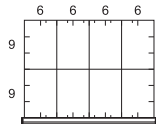
RONHF-A030404 8 COMPARTIMIENTOS
