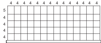
R__KE-A1356__ 70 COMPARTIMIENTOS
