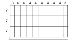
R_GE-A0920_ 30 COMPARTIMIENTOS
