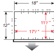
MEDIO CAJÓN LATERAL (FONDO CONTRA FONDO)
