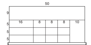
R_JG-C0508__ 14 COMPARTIMIENTOS
