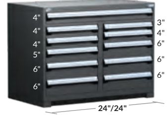
11 CAJONES R5KHE-3405 48" x 24" x 36" R5KHG-3405 48" x 27" x 36"
