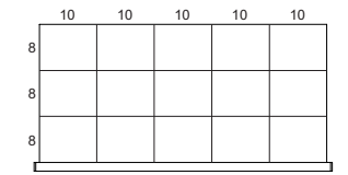
R_JG-A0410__ 15 COMPARTIMIENTOS
